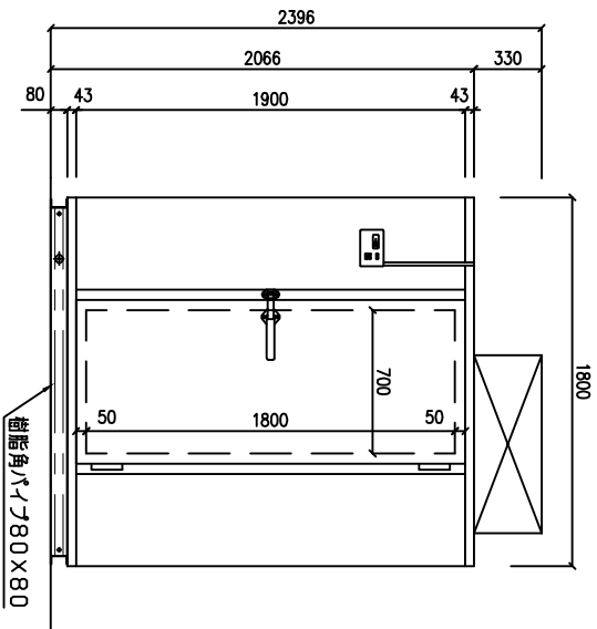
《 立面図 》
