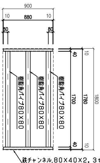
《 基礎図 》
