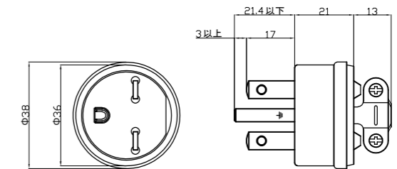
単相200Vプラグ形状 (接地極付 15A 250V)
